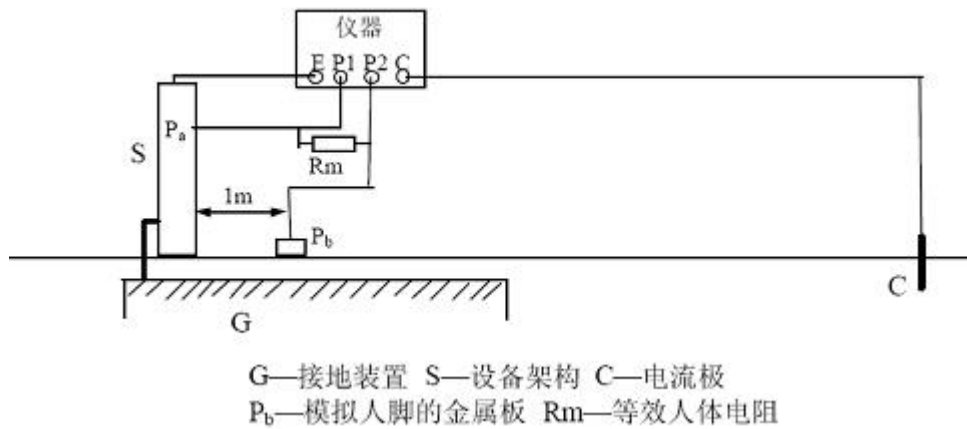
图5 接触电压测量接线图
