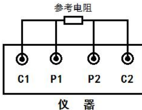
图 13 仪器自检接线图
