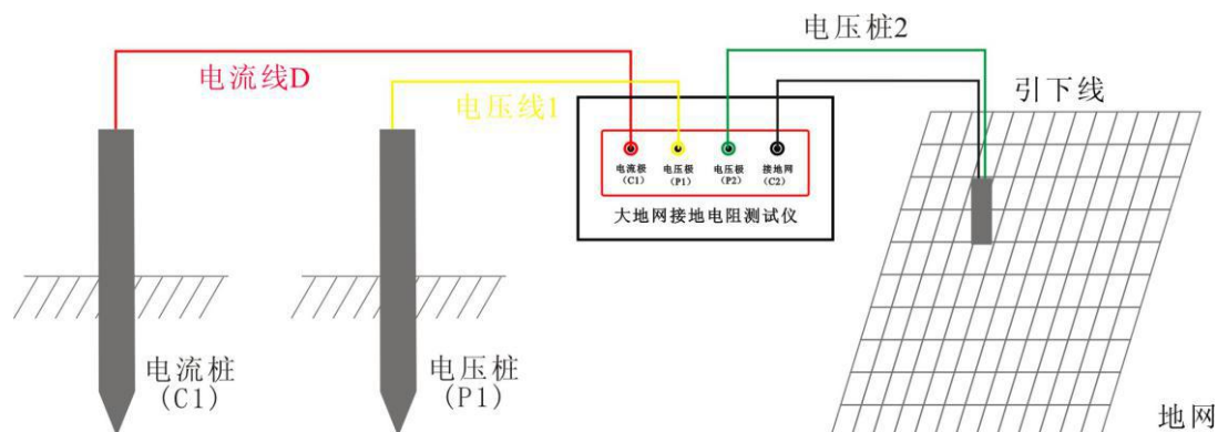
图4 四极法测量接线图
