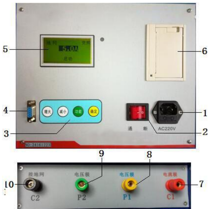
图 2 面板示意图
