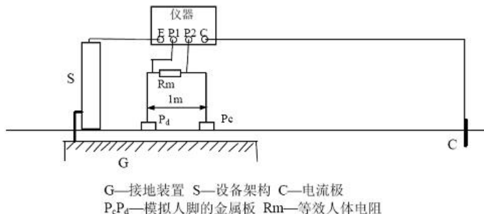
图6 跨步电压测量接线图
